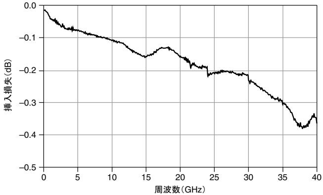
図 1. 標準挿入損失
